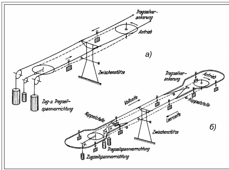
Рис. 52. Схема: а — взаимного расположения опоры, роликовых батарей и подвешенной платформы; б — устройства металлической несущей конструкции. Реконструкция автора
